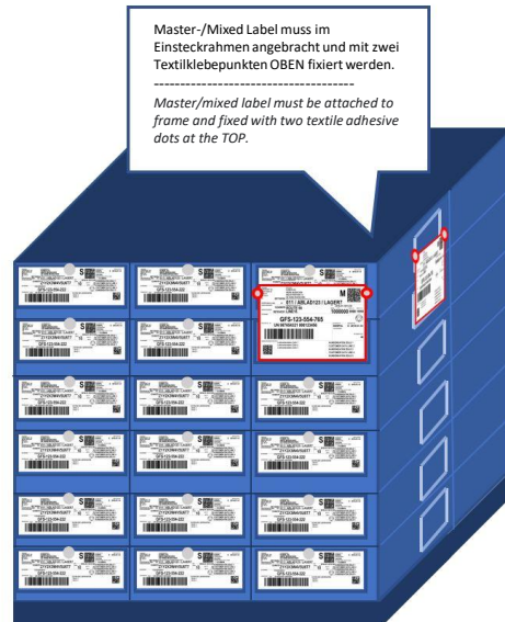
Gültig für 004147 / 006147 und allen KLTs mit gleichen Maßen Valid for 004147 / 006147 and all KLTs with the same dimensions
