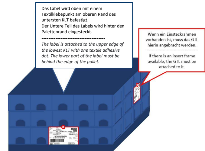
!!! SONDERFALL !!! SPECIAL CASE !!! Gültig für 003147 und allen KLTs mit gleichen Maßen Valid for KLT 003147 and all KLTs with the same dimensions
